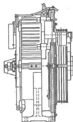
明電製 T3.5/5.2/6.8 (ギヤレスマシン)
